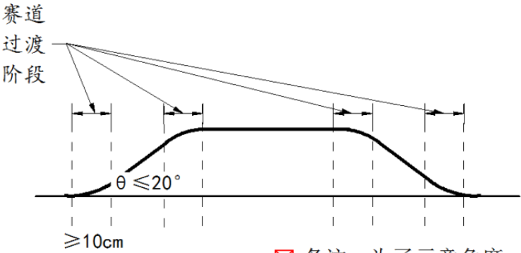
图 17 坡道示意图
