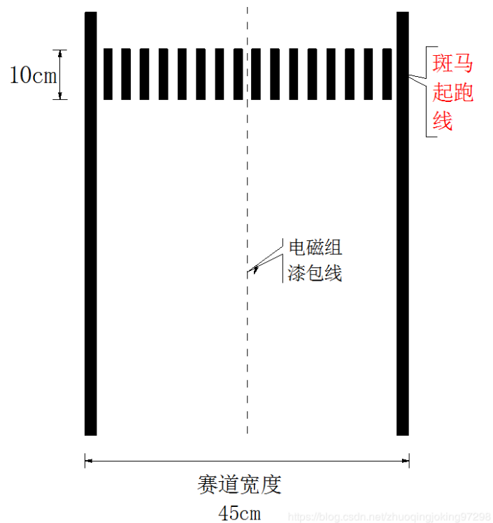
图 10 斑马起跑线
