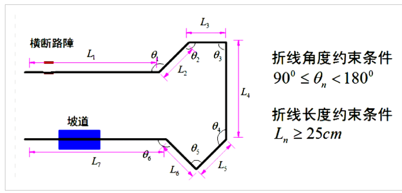
图 3 赛道折线几何参数
