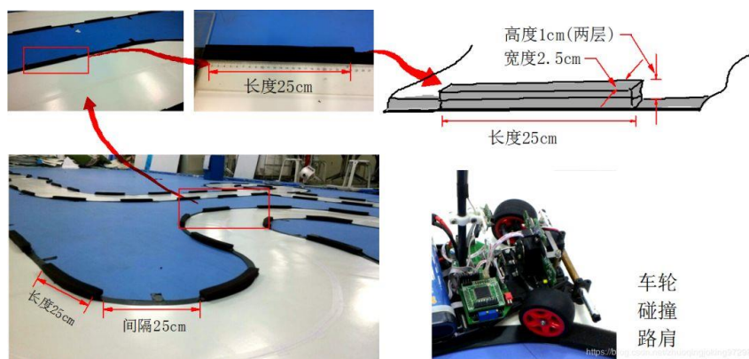
图 13 赛道路肩
